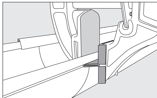
Klem tangen omkring tagrendens forvulst, indtil der lyder er "klik".
