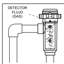
Instalación RECOMENDADA
