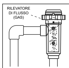
Installazione CONSIGLIATA
