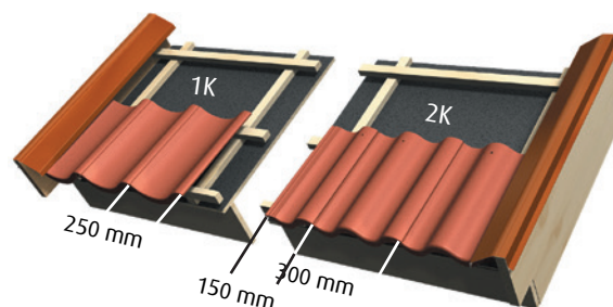
Figur 9. Opdel tagbredden i antal tagsten. Husk at den sidste sten ud mod ventre gavl dækker 330 mm for 2K og 280 mm for 1K.
