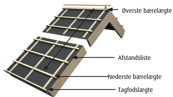
Figur 5. Udregn antallet af tagsten. Se også tabel 5.
