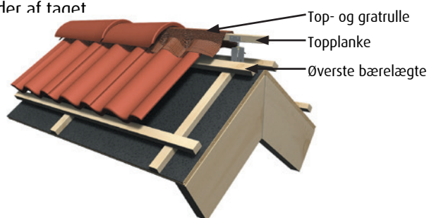
Figur 4. Afstanden fra topplankens centrum til øverste bærelægte skal være ca. 40 mm, se tabel 3. Afprøv, at rygningsternen overlapper øverste række tagsten på forsvarlig vis.
