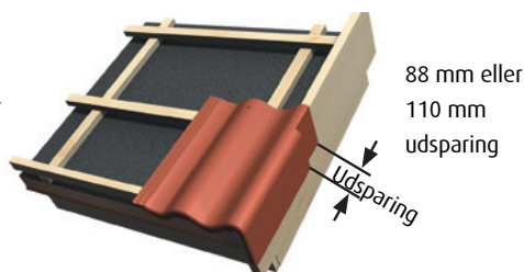
Figur 6. Benders vindskedesten giver en ekstrem stærk tætning.
