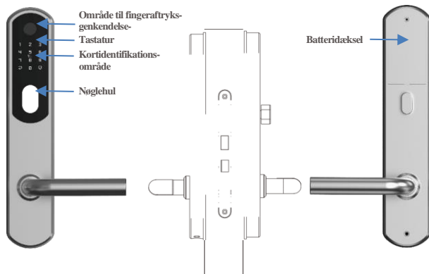
Udvendigt langskilt
